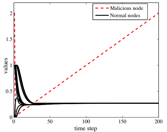
(b) W-MSR.
